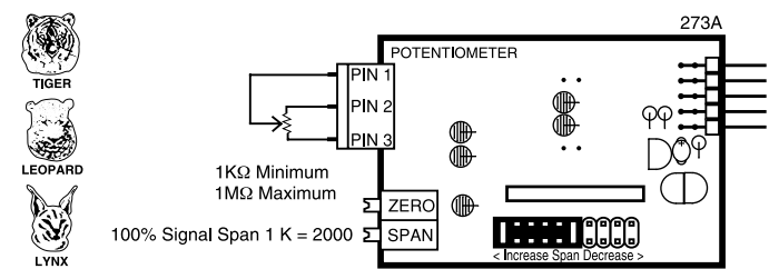
IR03: Linear Potentiometer 1KΩ min
