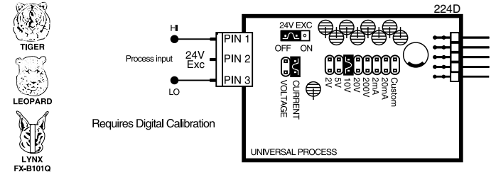
IR02: 3 wire Potentiometer 1KΩ min (0-F.S.)
